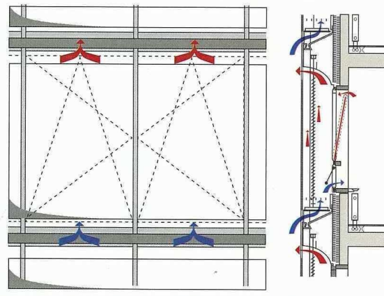
Figura 1 - Esempio di Box Window con sistema schermante integrato (Fonte: rivista Cda n. 07/08)
