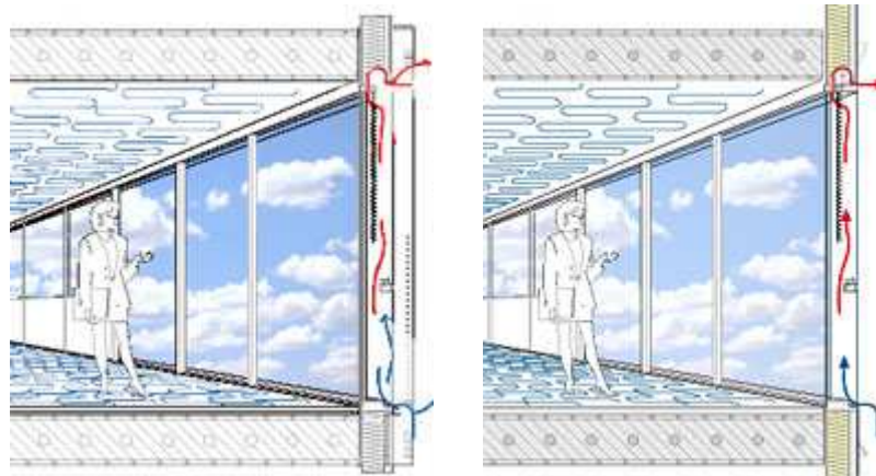
Figura 2 – Esempio di facciata ventilata naturalmente (a sinistra) e meccanicamente (a destra) con sistema schermante integrato nella doppia pelle (Fonte: [2])
