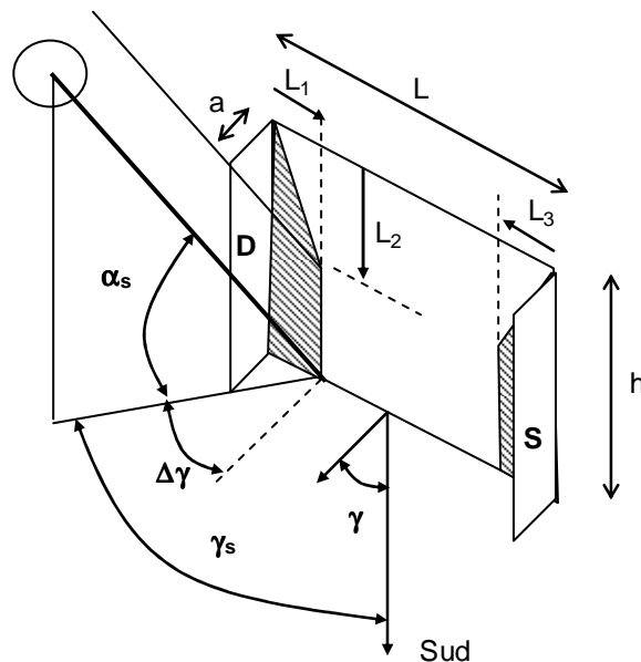
Figura 7 – Ombre proprie dovute a schermi verticali
